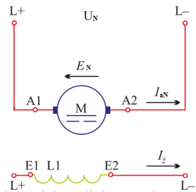
2 pav. Nepriklausomojo žadinimo elektros mašinos sujungimų schema: E_N – elektrovaros jėga; U_N – gnybtų įtampa; I_{aN} – inkaro grandinės srovė; I_z – žadinimo apvijos srovė
